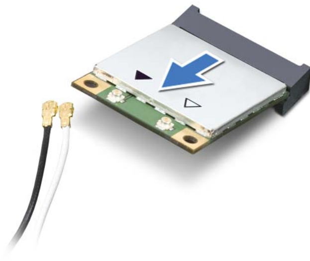
1 разъем мини-платы беспроводной сети 2 мини-плата беспроводной сети
